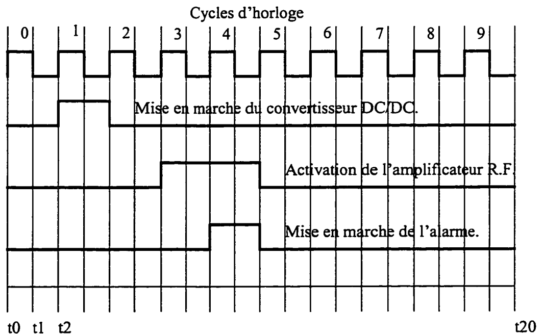
Figure 4.12. Les formes d'ondes des sorties du superviseur d'alimentation.
