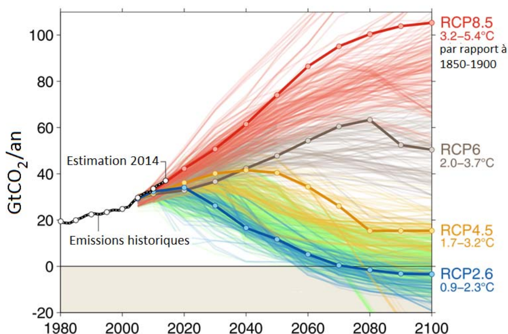
Figure 6 : émissions annuelles de dioxyde de carbone ( \text{CO}_2 ) dues à la combustion des combustibles fossiles et à la production de ciment exprimées en milliards de tonnes (Gt).
