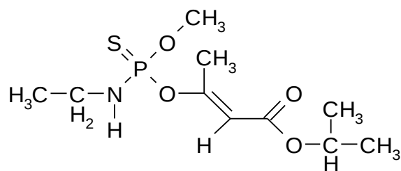
Propétamphos
