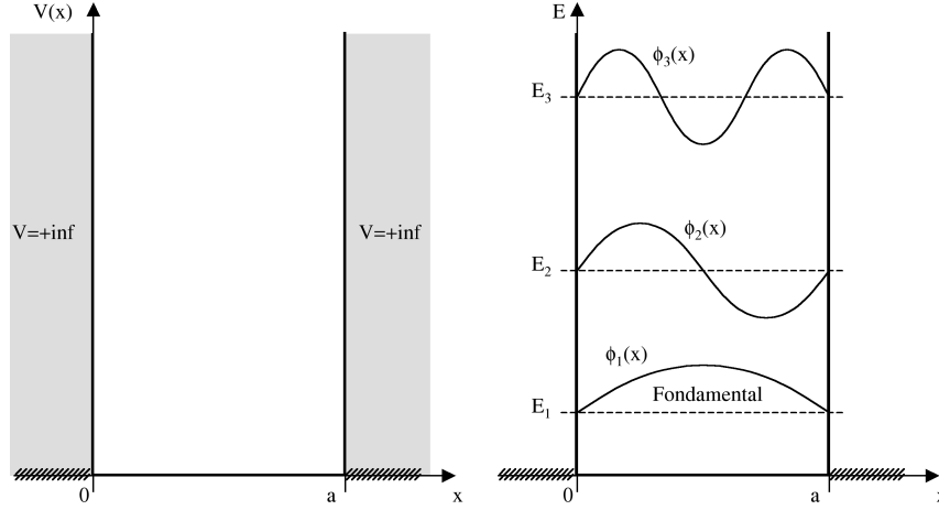
Fig. 10.1. Le puits de potentiel infini en dimension 1. À gauche : Représentation du champ de potentiel. Les parties grisées correspondent à V = +\infty . À droite : Les trois premiers niveaux d'énergie.
