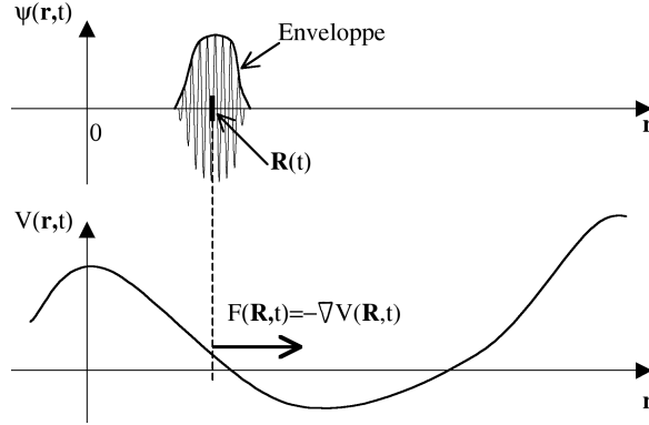
Fig. 9.1. La limite classique : lorsque le paquet d'onde est très piqué, l'accélération de sa position moyenne \mathbf{R}(t) s'identifie, au terme de masse près, à la dérivée locale du champ de potentiel.
