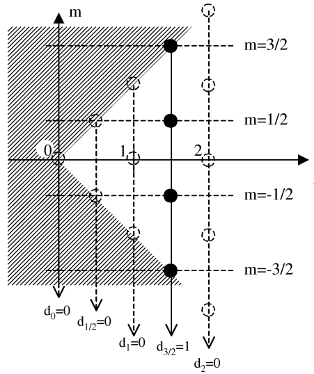
Fig. 12.10. Dimensions des sous espaces V_{j,m} dans l'exemple du spin de nombre I = \frac{3}{2} : seuls les 4 espaces pour lesquels j = \frac{3}{2} sont autorisés. Ils sont chacun de dimension 1.
