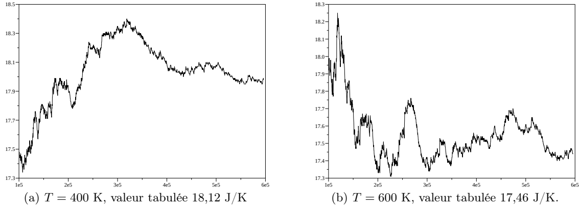
Fig. 5.9. Estimation de la capacité calorifique molaire à volume constant C_v en fonction du nombre de pas de temps.
