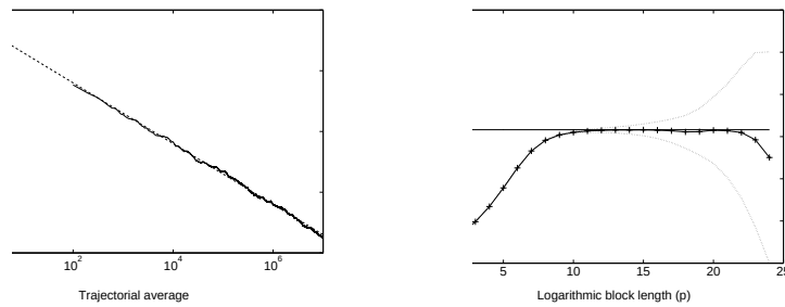
Fig. 5.6. Gauche : Variance \sigma_{N,M}^2 en fonction de la longueur N de la trajectoire, avec M = 100 trajectoires indépendantes. L'approximation linéaire (ligne en traits interrompus) donne \sigma_{N,M}^2 \simeq 40N^{-1} . Droite : Estimation de la déviation standard par moyenne par blocs, en fonction de la taille n = 2^p des blocs (ligne pleine). On a moyenné sur 100 estimations indépendantes (intervalle de confiance en traits pointillés).
