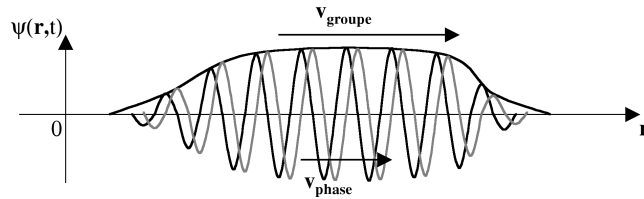
Fig. 8.4. Vitesse de phase et vitesse de groupe pour le paquet d'onde monochromatique étalé.
