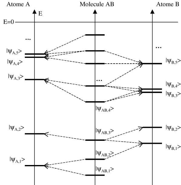
Fig. 14.2. L'approximation CLOA : les diagrammes énergétiques de l'atome A isolé, de la molécule AB , et de l'atome B isolé sont représentés de manière juxtaposée. On constate en pratique que chaque orbitale |\phi_{AB}\rangle de la molécule s'approxime comme une combinaison linéaire de niveaux atomiques énergétiquement proches, désignés par les flèches en pointillés. Par exemple, l'état noté |\phi_{AB,3}\rangle est quasiment exclusivement une combinaison linéaire de |\phi_{A,2}\rangle , |\phi_{B,1}\rangle et |\phi_{B,2}\rangle . Il ne s'agit ici que d'un dessin de principe. Des schémas plus précis sont donnés dans la suite du cours.
