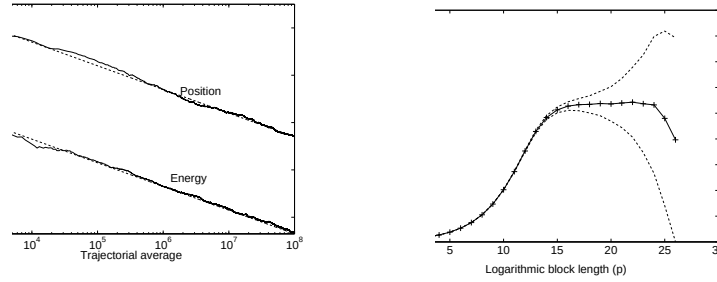
Fig. 5.7. Gauche : Variance \sigma_{N,M}^2 en fonction de la longueur N de la trajectoire, avec M = 100 trajectoires indépendantes. L'approximation linéaire (ligne en traits interrompus) donne \sigma^2 \simeq 2500 pour l'observable position, et \sigma^2 \simeq 0.20 pour l'observable énergie potentielle. Droite : Estimation de la déviation standard par moyenne par blocs, en fonction de la taille n = 2^p des blocs (ligne pleine), pour l'observable position. On a moyenné sur 100 estimations indépendantes (intervalle de confiance en traits pointillés). La valeur estimée de la variance est \sigma^2 \simeq 2800 .
