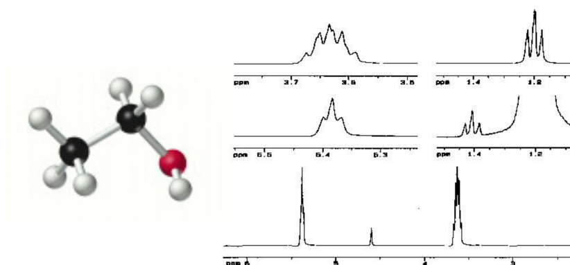
Fig. 10.12. Spectres de résonance magnétique nucléaire (RMN) de la molécule d'éthanol \text{CH}_3\text{-CH}_2\text{-OH} . En RMN, le système quantique étudié évolue sur un nombre fini d'états quantifiés. Le spectre ne possède ainsi qu'un nombre fini de raies.
