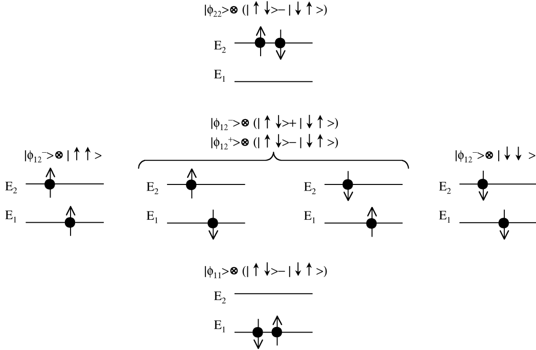
Fig. 13.8. Les 6 diagrammes énergétiques qui peuvent être construits pour deux fermions de spin \frac{1}{2} placés sur un système à deux niveaux. Quatre de ces diagrammes sont directement identifiables aux états de base |22\rangle \otimes |\uparrow\downarrow\rangle , |12^-\rangle \otimes |\uparrow\uparrow\rangle , |12^-\rangle \otimes |\downarrow\downarrow\rangle et |11\rangle \otimes |\uparrow\downarrow\rangle . L'identification avec les états |12^+\rangle \otimes |\uparrow\downarrow\rangle et |12^-\rangle \otimes |\uparrow\downarrow^+\rangle est plus délicate. C'est là une limite de ce système de représentation graphique (la vérité étant dans la forme mathématique des états).
