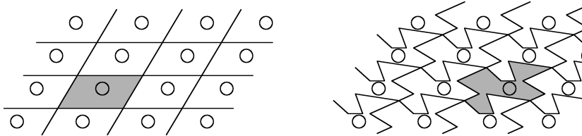
Fig. 14.14. Différents choix possibles de cellule unité pour un même réseau bi-dimensionnel. Le choix d'une cellule de forme simple (à gauche) est une commodité pratique, mais pas une obligation.
