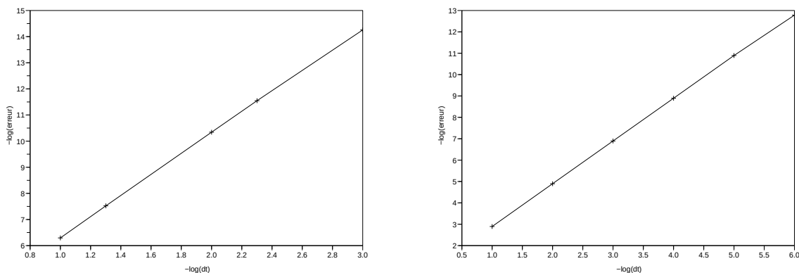
Fig. 3.3. À gauche : tracé de -\log(e_T(\Delta t)) en fonction de -\log(\Delta t) pour le schéma de Runge-Kutta d'ordre 4 dans le cas de l'oscillateur harmonique. À droite : cas du schéma de Störmer-Verlet.
