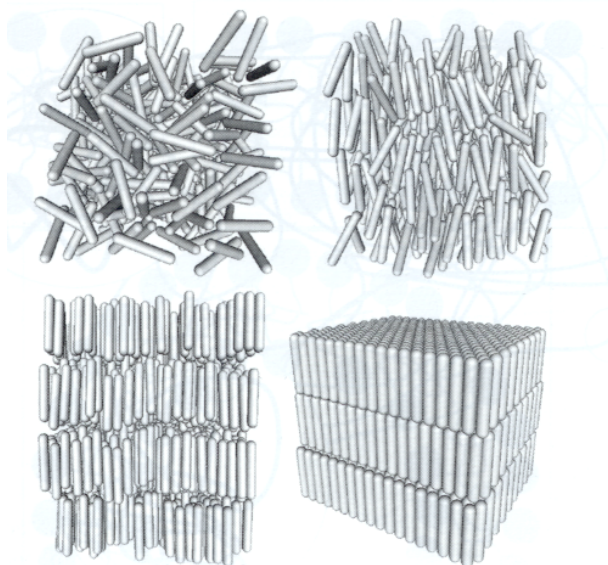
Fig. 1.5. Différentes phases des « sphérocyindres » durs (cylindres fermés par deux hémisphères) : de gauche à droite et de haut en bas, phases isotrope, nématique, smectique, cristalline.
