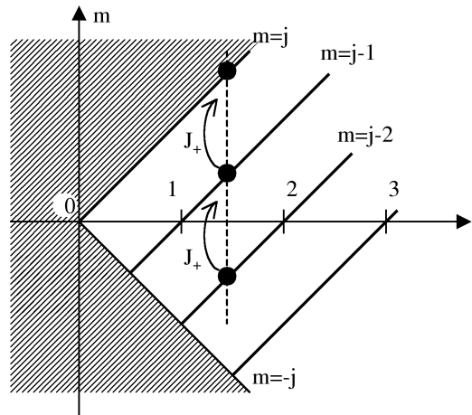
Fig. 12.5. Etape 3 de la démonstration : Action de l'opérateur \hat{J}_+ sur les couples de valeurs (j, m) . Les seules zones restant autorisées pour ces valeurs sont les demi-droites m = j - \text{entier} ( m \geq -j ).
