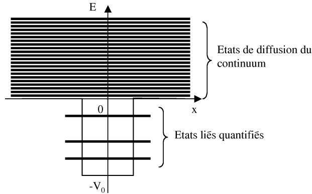
Fig. 10.9. Structure du spectre énergétique complet du trou de potentiel à une dimension. Les énergies négatives sont quantifiées. Les énergies positives sont toutes accessibles, et forment un continuum d'états de diffusion. Cette structure est à rapprocher de celle du spectre énergétique du potentiel Coulombien.
