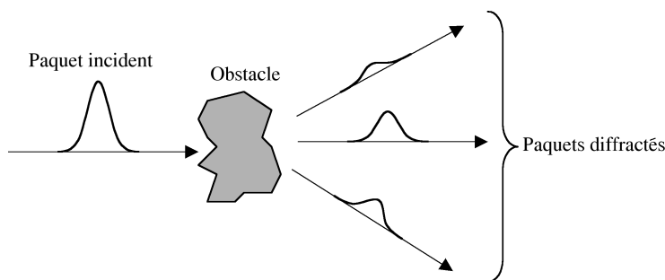
Fig. 8.7. 'Eclatement' d'un paquet d'onde en une superposition de trois paquets indépendants lors de sa diffraction sur un obstacle. Après l'impact, la particule se trouve simultanément répartie dans les trois paquets diffractés.
