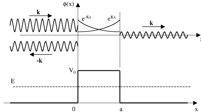
Fig. 9.3. Les cinq composantes des états stationnaires d'énergie E < V_0 correspondant à une particule arrivant sur la barrière par la gauche.
